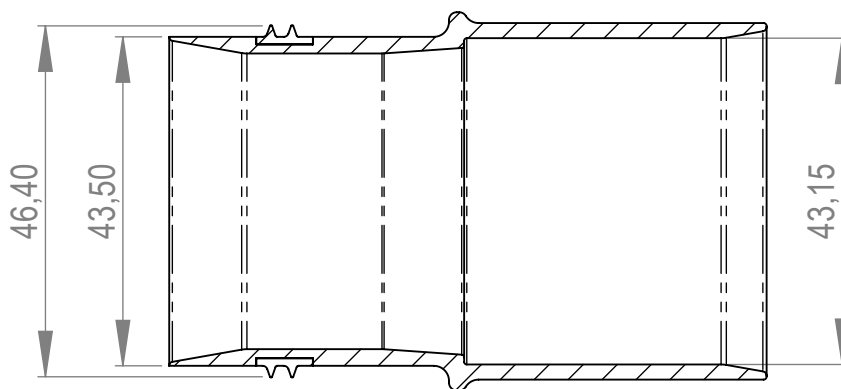
A-A (1 : 1)
