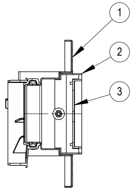
A-A (1 : 3)
