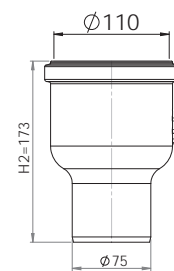
Brunnsdel Bottenutlopp Ø75
