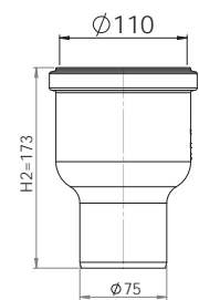
Brunnsdel Bottenutlopp Ø75
