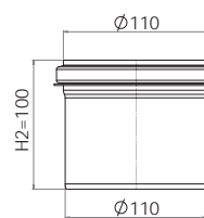
Brunnsdel Bottenutlopp Ø110
