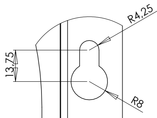
DETALJ A SKALA 1 : 1
